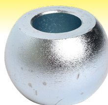
2539 Lower Link Ball Cat 3/2 ID 29 OD 63.5
