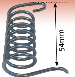
PZ100 PZ Hay Bob Spring RH
